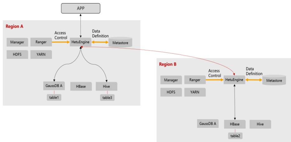
图9-8 HetuEngine 跨域功能示意
