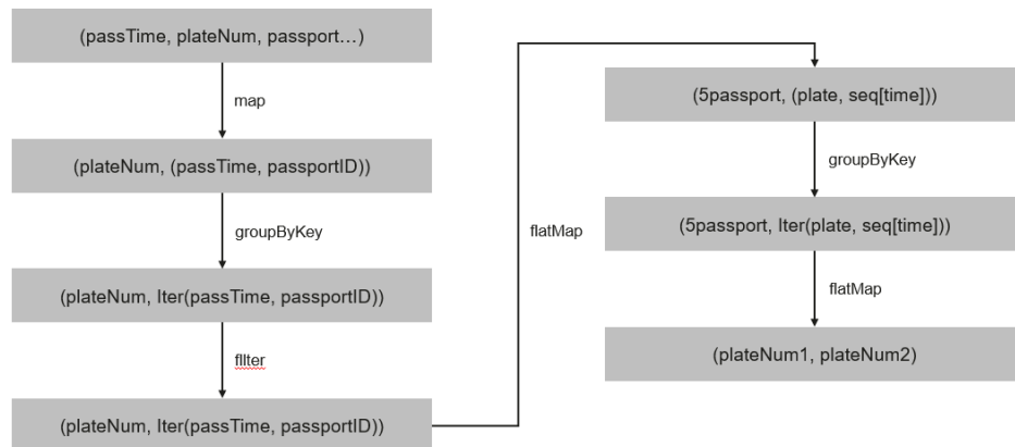
图19-7 实现 2 逻辑
