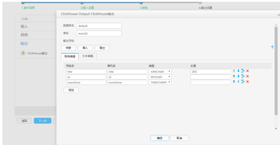
图15-39 算子输出
