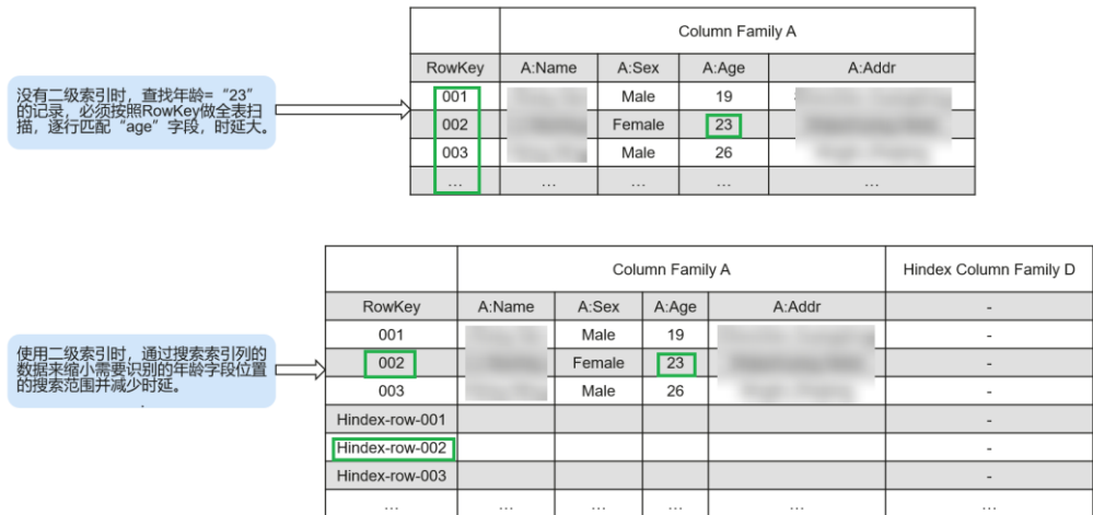
图7-2 HBase HIndex
