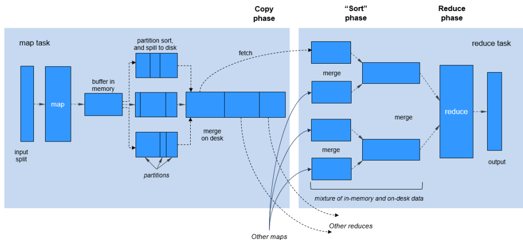
图16-2 Shuffle 过程
