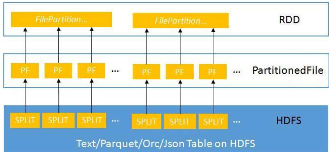
图19-8 小文件合并
