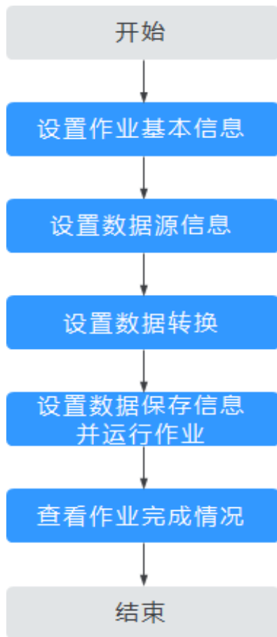
图15-45 导出流程示意
