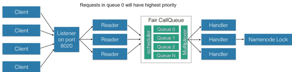
图8-5 基于 FAIRCallQueue 的 NameNode 请求处理
