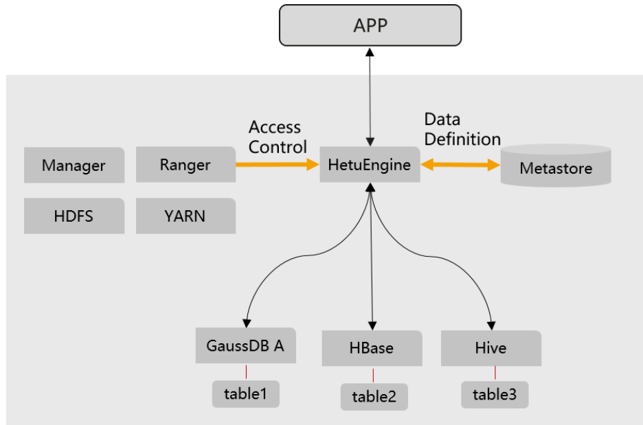
图9-7 HetuEngine 跨源功能示意
