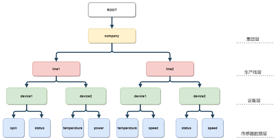
图13-1 数据结构
