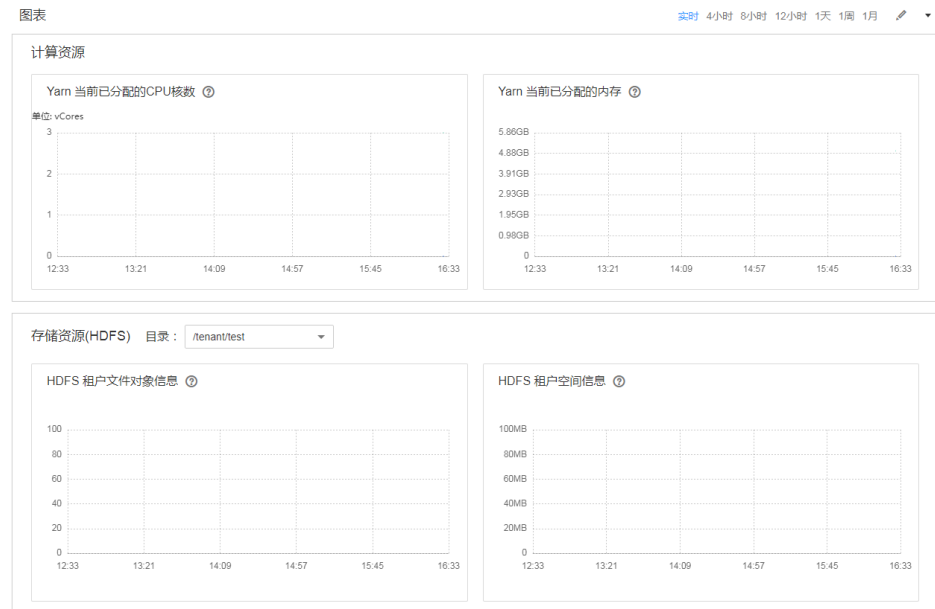
图8-17 精细化监控
