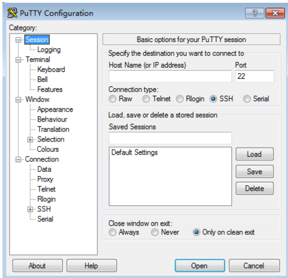
图3-2 单击 Session
