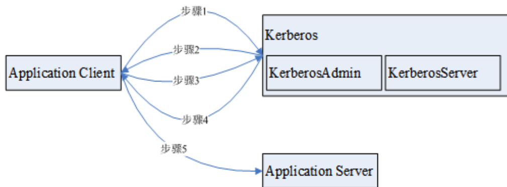
图10-1 原理架构
