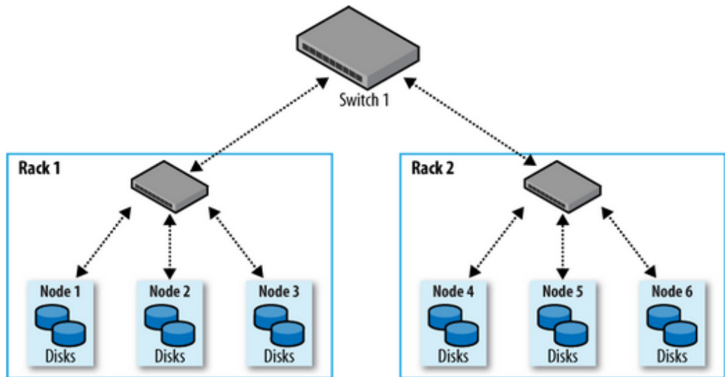
图8-6 两层网络结构
