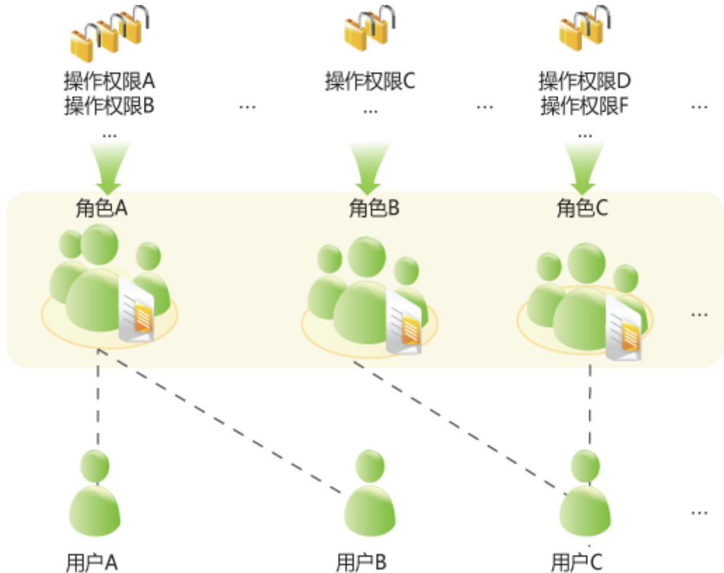
图8-24 权限模型
