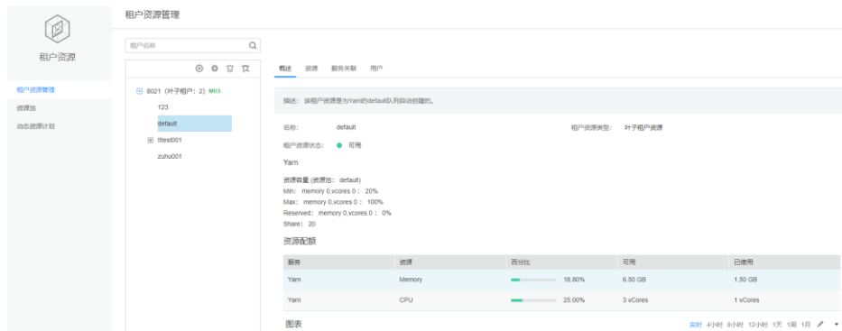
图8-16 多租户管理
