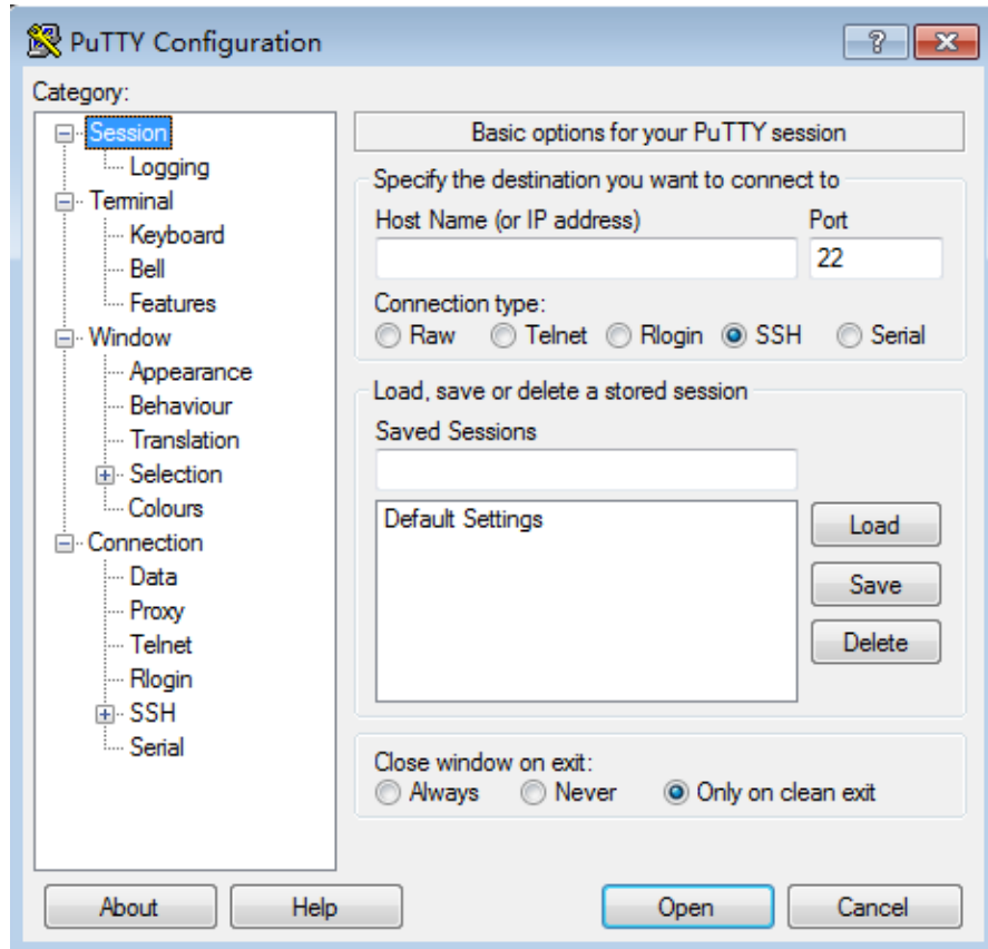
图3-1 单击“Session”
