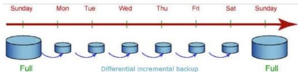
图10-2 快照备份过程
