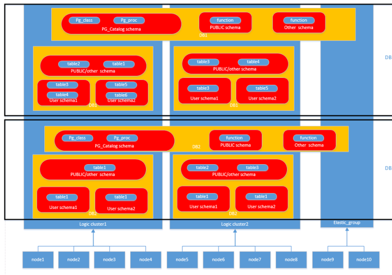
图15-1 逻辑集群、数据库、表层次关系
