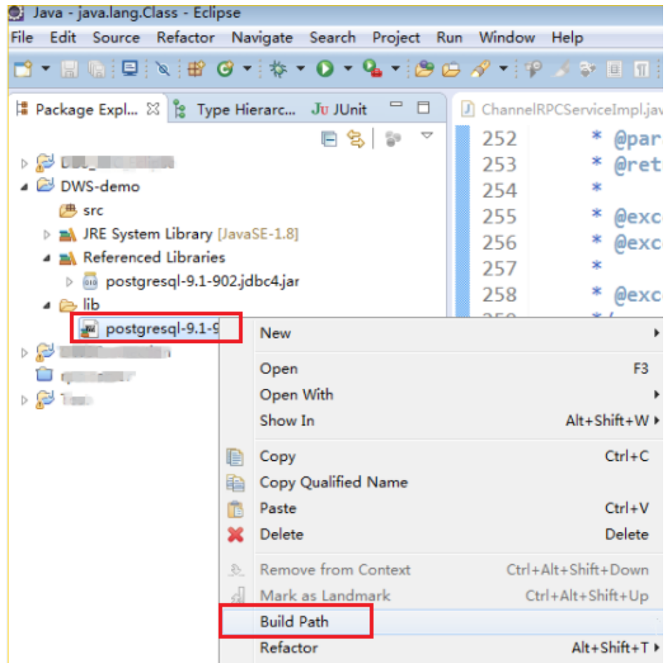
图6-6 引用 jar 包
