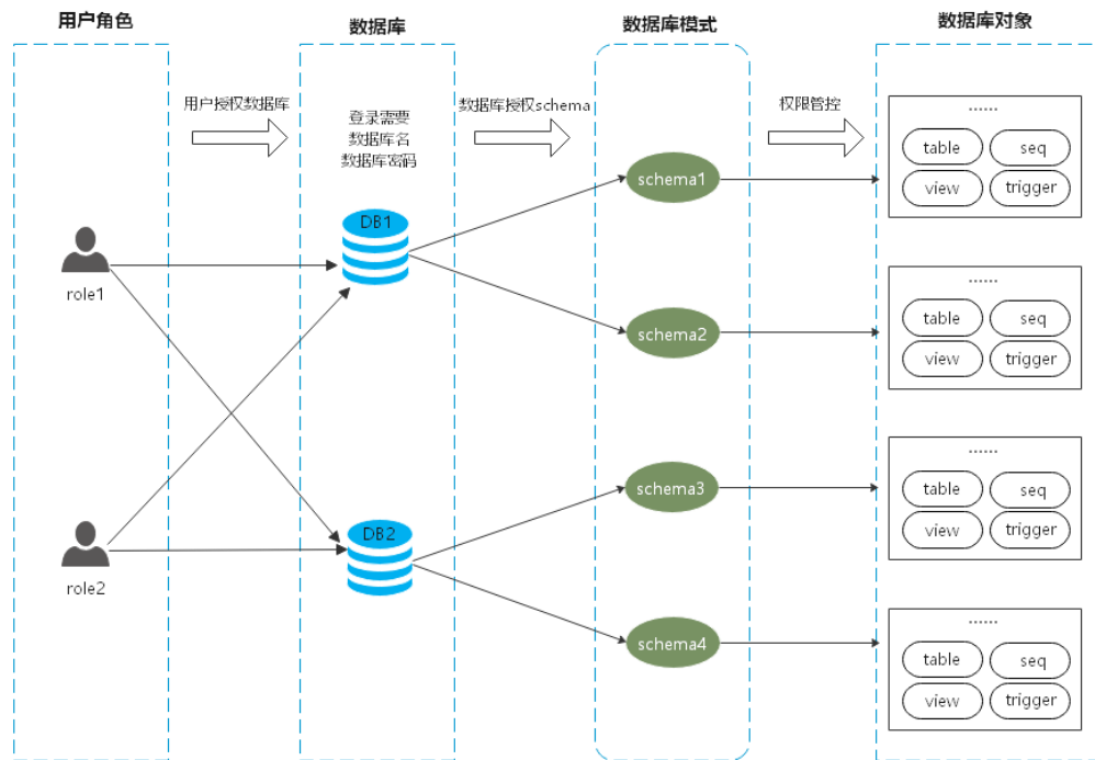
图16-3 权限控制
