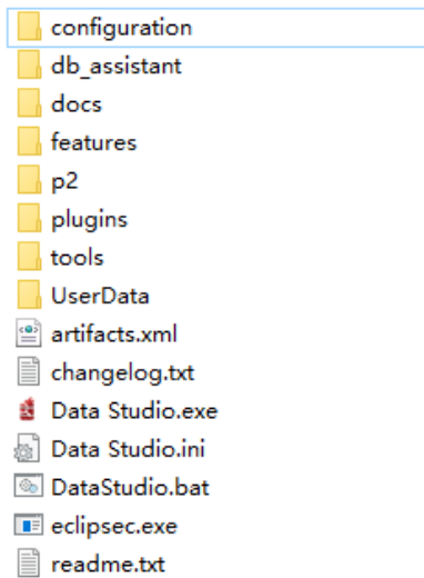
图6-2 启动客户端
