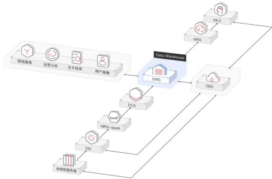
图1-5 电商场景
