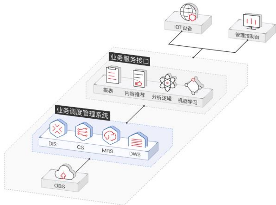
图1-6 IoT 场景
