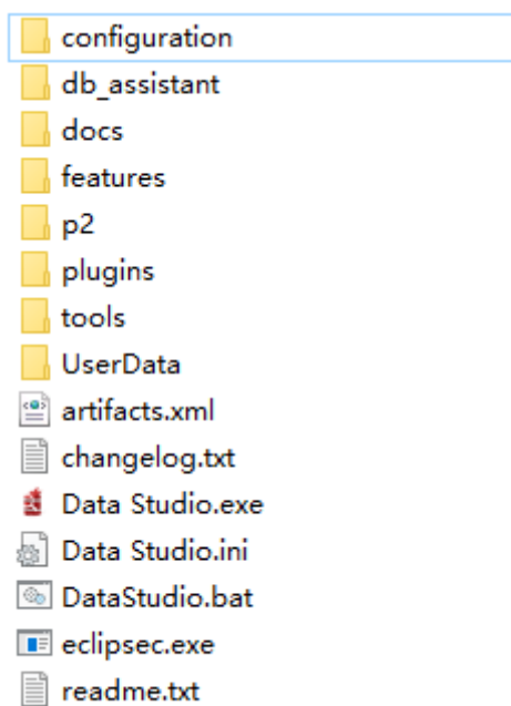
图2-2 启动客户端
