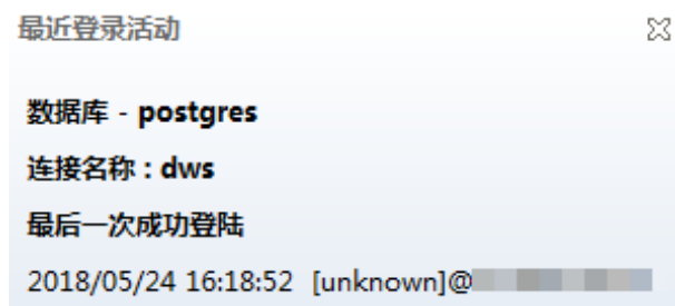
图2-5 登录成功
