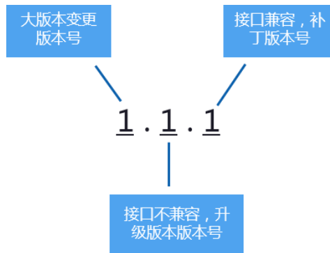
图9-1 版本说明
